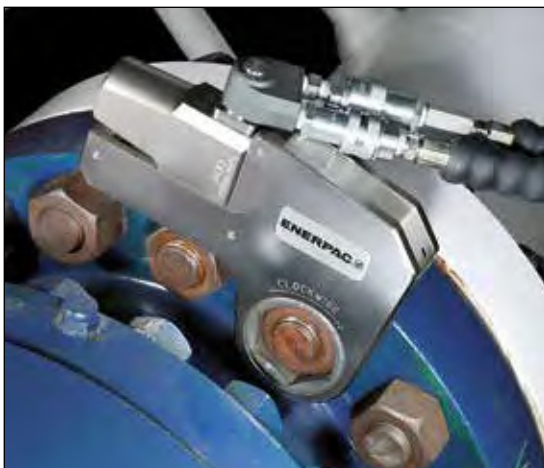
◀ Las bombas para llaves dinamométricas de la series ZE4T son idóneas para esta llave W2000X.
