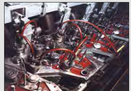
▲ Tuercas hidráulicas en un motor diesel.
