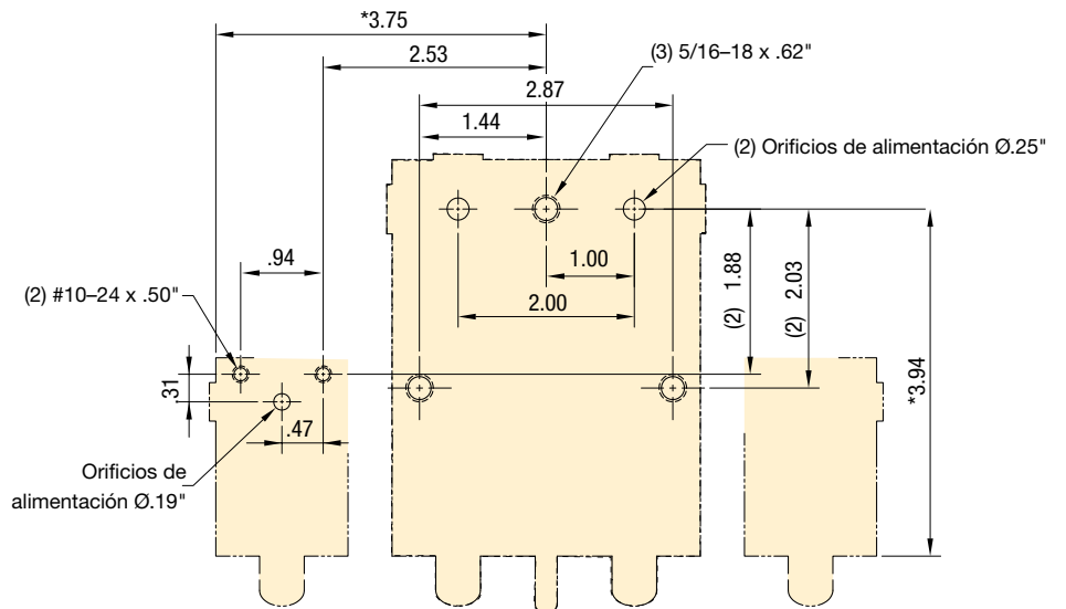
MCR-21 con MCRA-11
