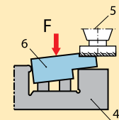
Figura 5b Pieza de trabajo posicionada incorrectamente
