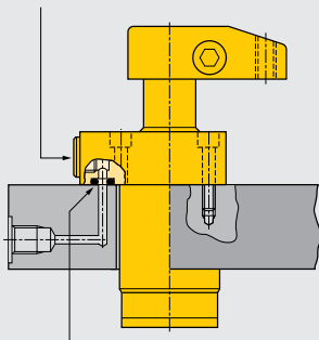
Orificio integrado con junta tórica
