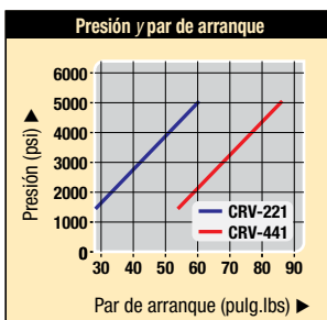
Pérdida de aceite del CRV-221=1,22 pulg 3 /min (20 cm 3 /min), CRV-441=2,44 pulg 3 /min (40 cm 3 /min)
