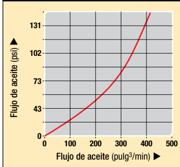
Flujo de aceite y caída de presión
