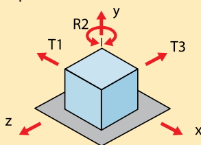
Figura 2 Cuerpo tridimensional
