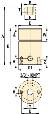
otros modelos RWH
