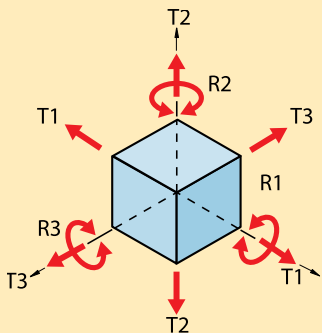
Figura 2 Cuerpo tridimensional
