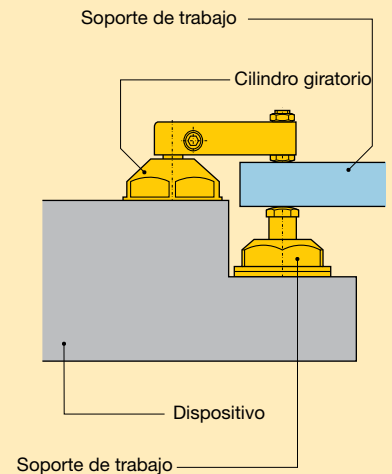
Figura 1 Uso combinado de cilindros de sujeción y soportes de trabajo.
