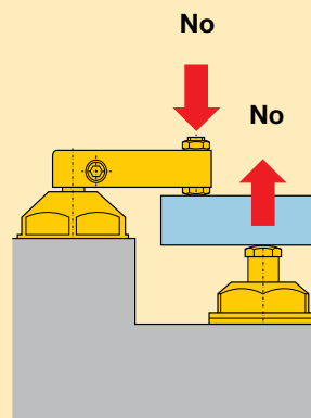
Figura 3 Una carga descentrada curvará la pieza de trabajo y producirá una deflexión fuera de control (Figura 3).
