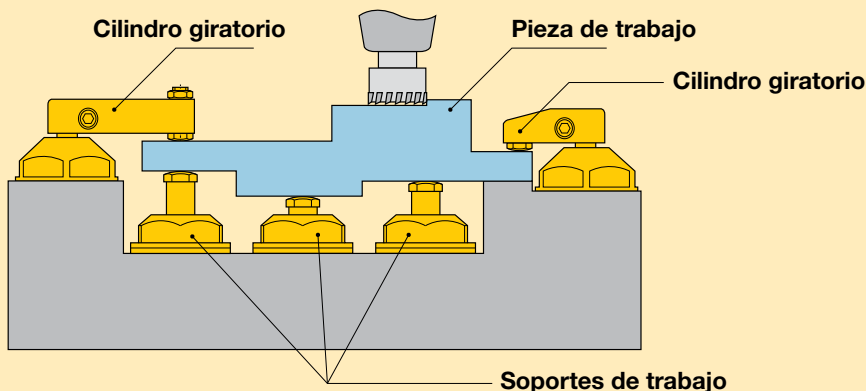
Figura 4 Los cilindros giratorios y los soportes de trabajo con avance por medios hidráulicos son muy sensibles al flujo de aceite aplicado. Para asegurar un funcionamiento seguro y confiable de dichos elementos, no se debe superar el caudal máximo de aceite que se indica en las páginas del catálogo y en las instrucciones. Si existen riesgos de caudales elevados de aceite, se recomienda utilizar válvulas de control de flujo para corregirlos.
