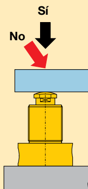
Figura 2 Para lograr resultados óptimos en la sujeción y repetibilidad de calidad, la dirección de la fuerza de sujeción debe ser axial en el eje longitudinal del émbolo del soporte de trabajo. Para asegurar un funcionamiento confiable y seguro, no se debe cargar lateralmente el soporte para piezas (Figura 2).
