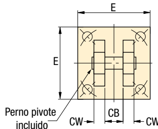
modelos TRCM Montaje en horquilla
