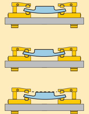
Figura 10b Elimine deformaciones mediante la utilización de soportes de bolas
