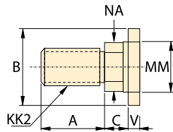
modelos TRFM Montaje de pie
