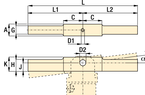
Modelos CAPT Brazos en "T" (únicamente para sujeción giratorios SU, SL, ST y SC)
