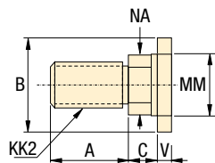
modelos TRFL Montaje en brida
