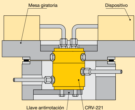
Pérdida de aceite del CRV-221=1,22 pulg 3 /min (20 cm 3 /min), CRV-441=2,44 pulg 3 /min (40 cm 3 /min)
