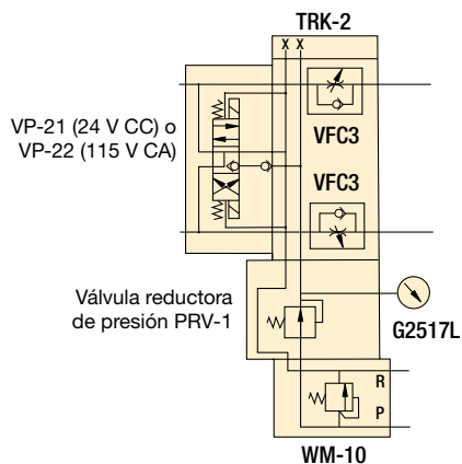
Ejemplo de un grupo de válvulas
