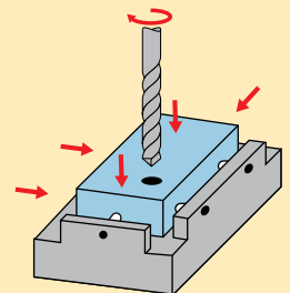
Figura 4c Pieza de trabajo totalmente limitada
